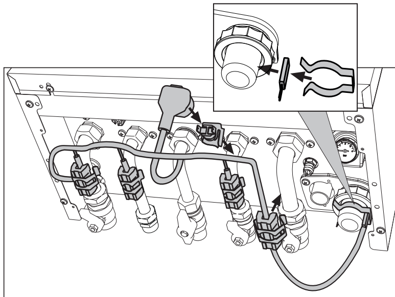
ΕΙΚ. 49- Κιτ προστασίας από τον παγετό
