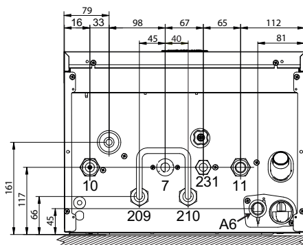
fig. 73- Vista inferior
