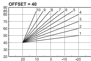
ΕΙΚ. 25- Παράδειγμα παράλληλης μετατόπισης των καμπυλών αντιστάθμισης
