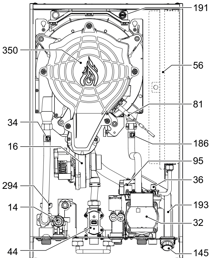
εικ. 75- Γενική όψη
