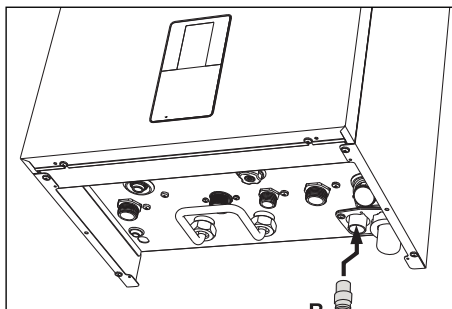
ΕΙΚ. 52- Σύνδεση εξαγωγής συμπυκνώματος
