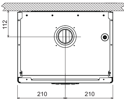
εικ. 73- Κάτωψη
