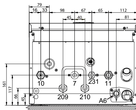
εικ. 74- Άνωψη
