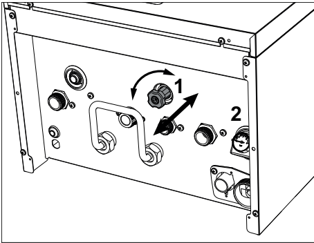
fig. 26- Filling knob
