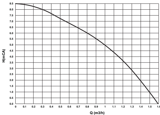
εικ. 79- Διαθέσιμο υπολειπόμενο μανομετρικό ύψος στην εγκατάσταση
