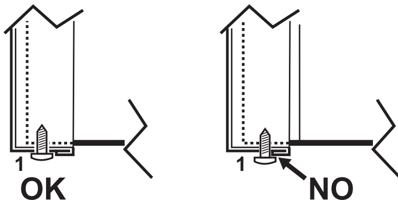
εικ. 57- Σωστή τοποθέτηση μπροστινού πίνακα
