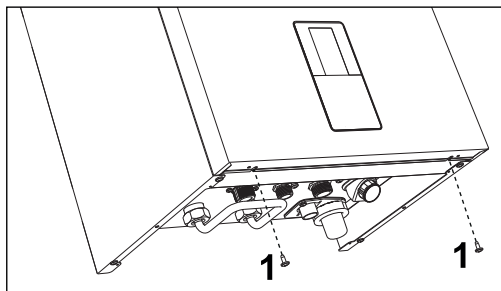
εικ. 56- Ανοιγμα μπροστινού πινάκα
