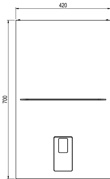
fig. 70- Vedere frontală
