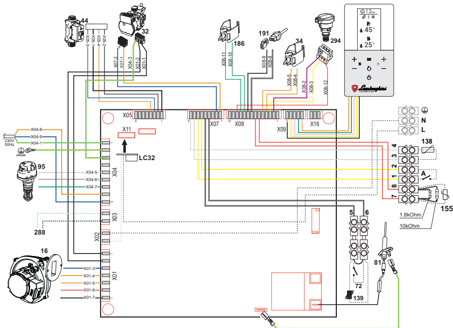
εικ. 80- Ηλεκτρολογικό διάγραμμα
