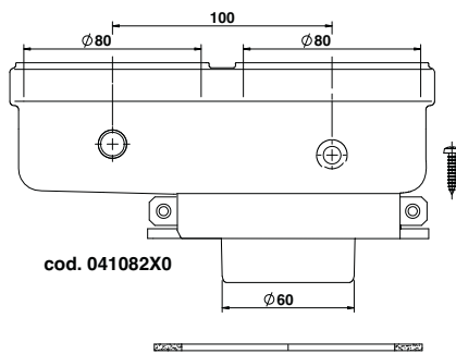
fig. 36- Accesorio inicial para conductos separados
