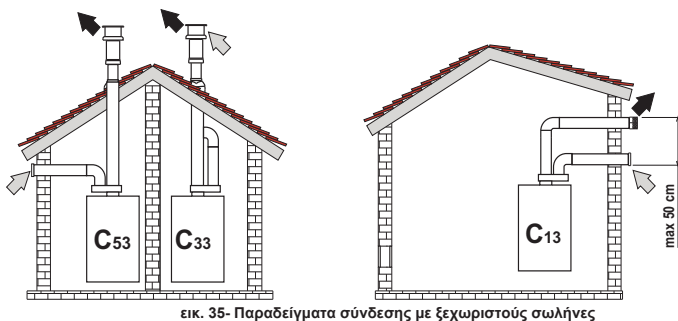
ΕΙΚ. 35- Παραδείγματα σύνδεσης με ξεχωριστούς σωλήνες
