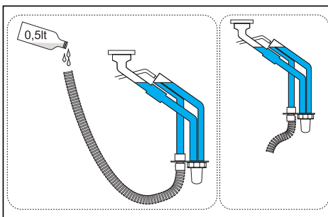
ΕΙΚ. 52- Σύνδεση εξαγωγής συμπυκνώματος
