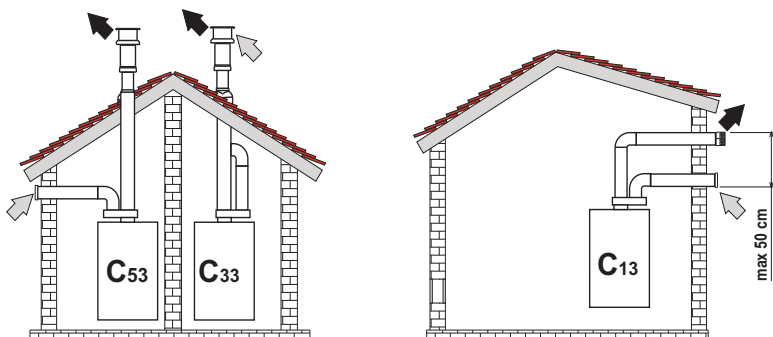
fig. 35- Ejemplos de conexión con tubos separados
