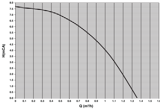
εικ. 78- Διαθέσιμο υπολειπόμενο μανομετρικό ύψος στην εγκατάσταση
