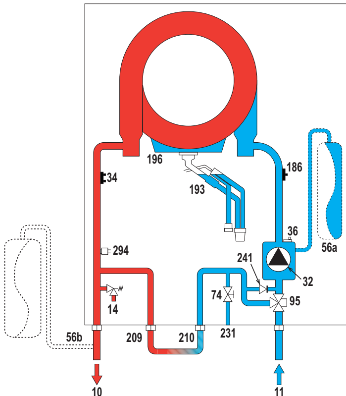
εικ. 76- Υδραυλικό κύκλωμα
