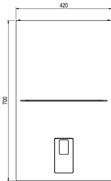
εικ. 71- Μπροστινή όψη
